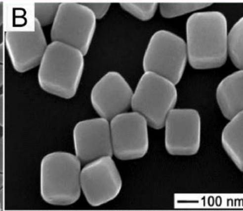
nanocubes
