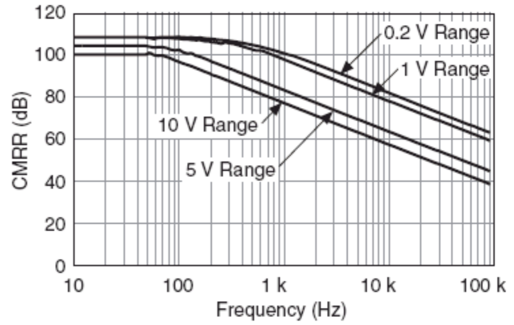
AI <0..79> CMRR
